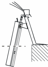
ESSMANN Lichtkuppel mit Konsole für einen 300 mm Hub ESSMANN Motoröffner.
